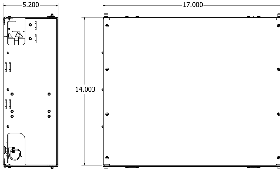
Dimensiones en pulgadas
